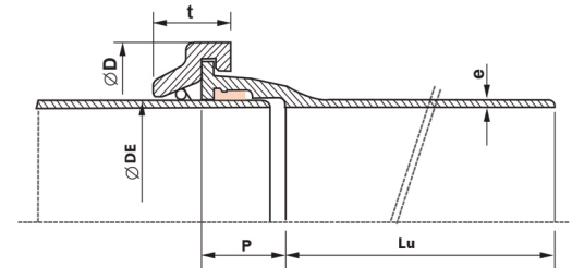
لوله با اتصال مقاوم در برابر لرزه R.J Pipe مطابق استاندارد ISO 2531:2009 C Class
