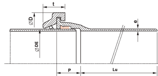
لوله با اتصال مقاوم در برابر لرزه R.J.Pipe مطابق استاندارد EN 545:2010 C Class
