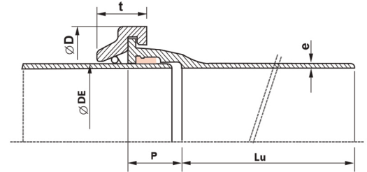
لوله با اتصال مقاوم در برابر لرزه R.J Pipe مطابق استاندارد ISO 2531:1998 K Class
