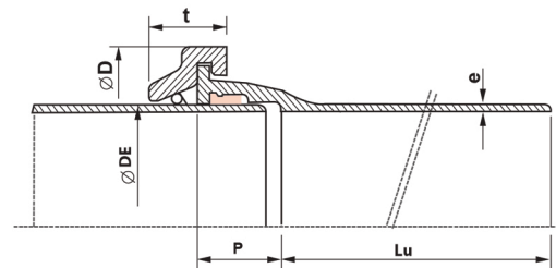
لوله با اتصال مقاوم در برابر لرزه R.J.Pipe مطابق استاندارد EN 545:2007 K Class
