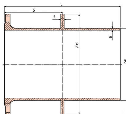
لوله چدن نشکن پادل دار یک سر فلنج یک سر اسپیکات
